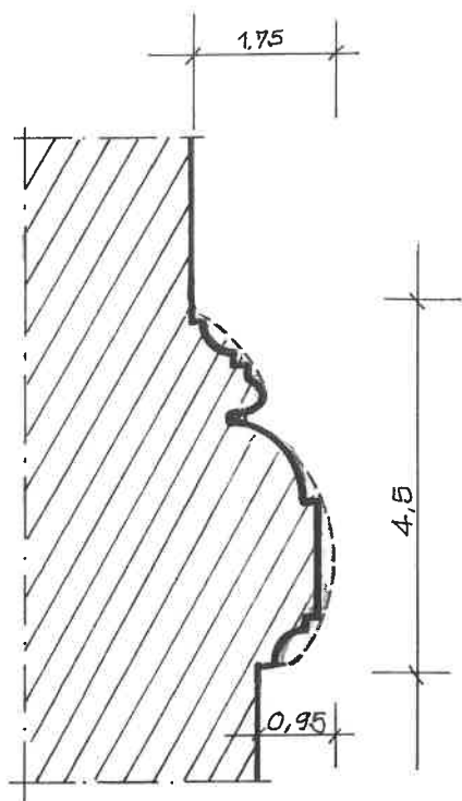
COUPE EF
