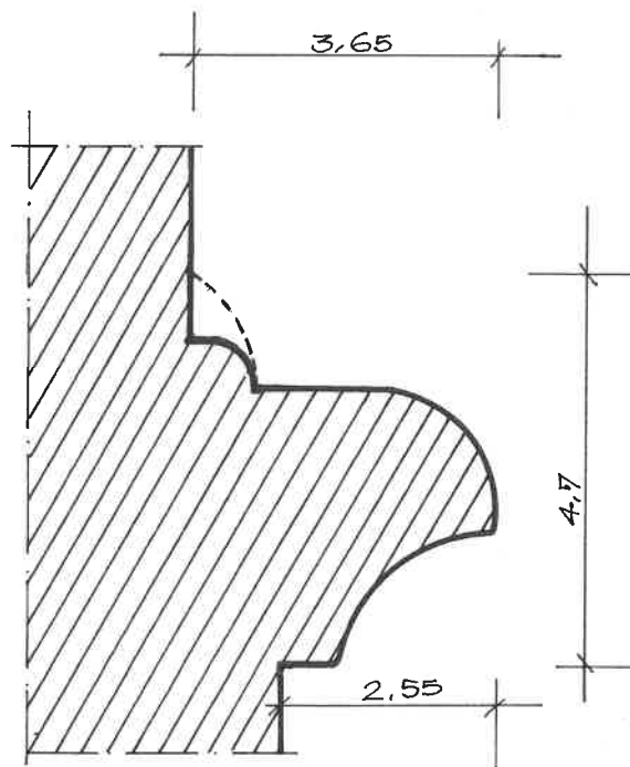
COUPE GH
